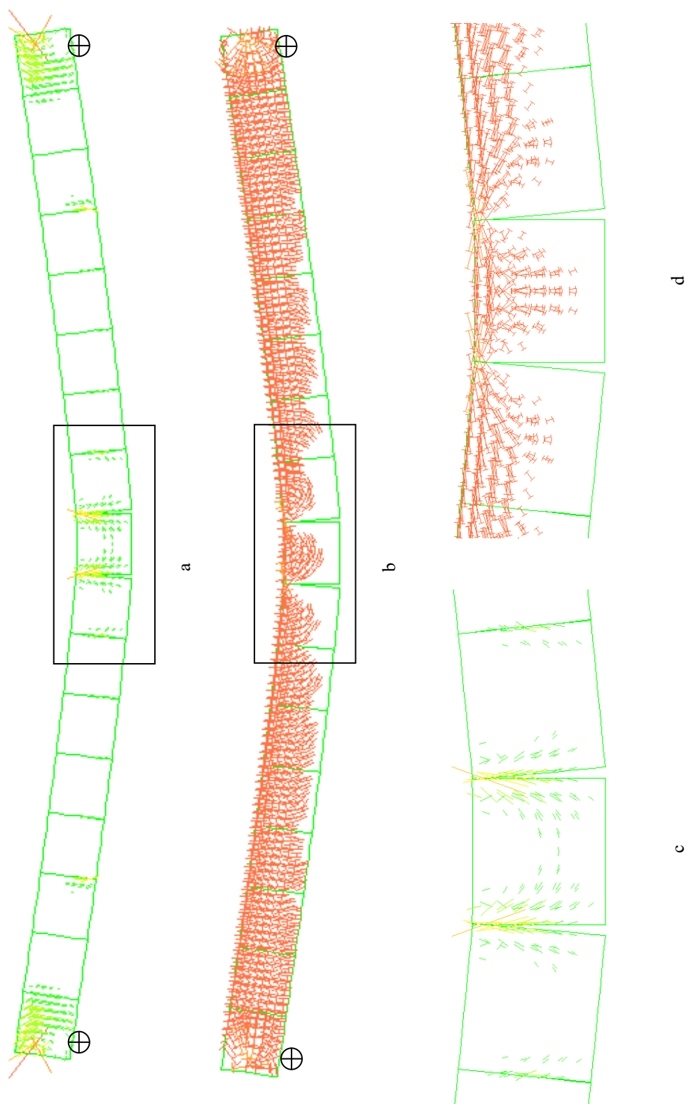
Figura 24. Campo de tensiones previo a la rotura por flexión obtenido en el ensayo numérico del puente isostático. ( \gamma_q=1,90 ). a) Tensiones principales de tracción ( |\sigma_I| \geq 2,0 \text{ MPa} ); b) Tensiones principales de compresión ( |\sigma_{II}| \geq 2,5 \text{ MPa} ); c) Detalle dodela central. Tensiones principales de tracción ( |\sigma_I| \geq 2,0 \text{ MPa} ); d) Detalle dodela central. Tensiones principales de compresión. ( |\sigma_{II}| \geq 2,5 \text{ MPa} ).
