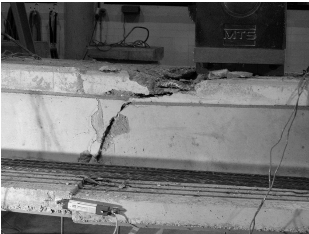
Figura 17. Ensayo V1-PC-70. Fase de prerrotura (a) y rotura (b)
