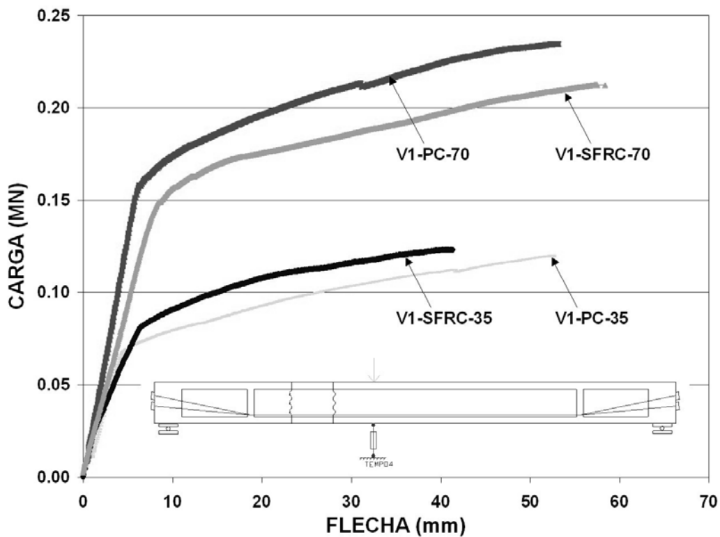
Figura 16. Gráfico carga-flecha bajo carga en ensayos V1
