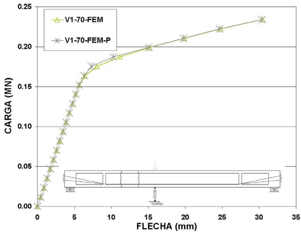
Figura 22. Curvas carga-flecha V1-70. Comparación de los resultados obtenidos con distintos modelos.
