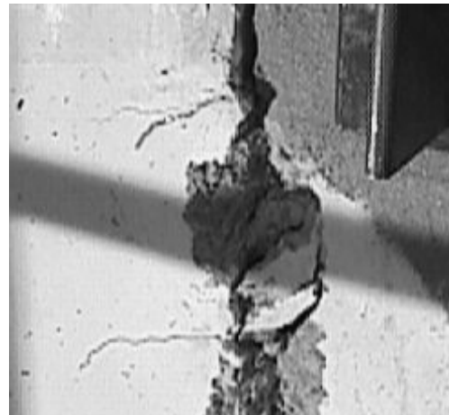
Figura 9. Detalle de la rotura de una llave PC-C.
