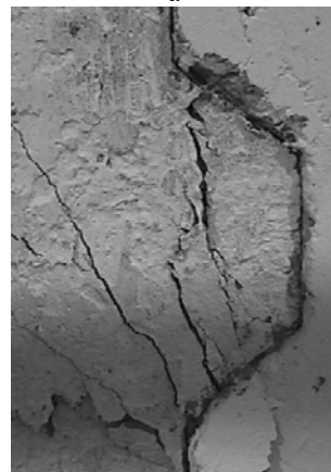
Figura 13. Fisuración en las llaves en los ensayos de junta abierta. a) flexión local b) cortante
