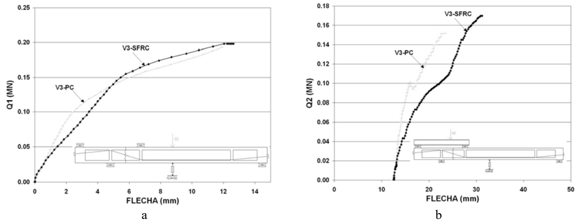
Figura 19.a. Gráfico carga Q1 -flecha en ensayos V3
