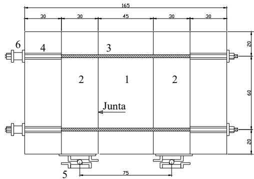
Dimensiones en cm
