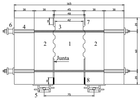
Dimensiones en cm
