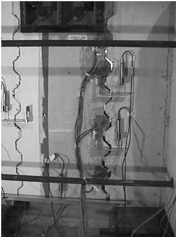
Figura 12. Desarrollo del ensayo PC-JA.
