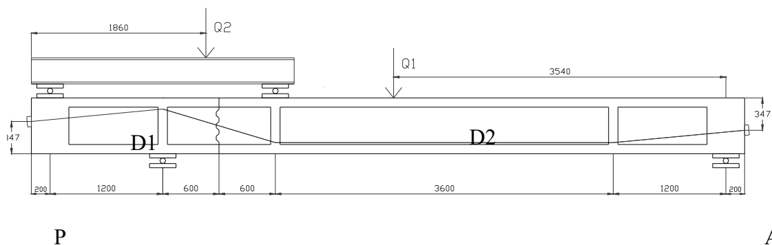
Figura 15. Configuración de la serie de ensayos V3. Dimensiones en mm.
