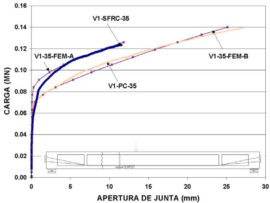
Figura 21. Curvas carga-apertura de junta en V1-35. Ensayos (V1-PC-35 y V1-SFRC-35) y análisis numérico (V1-35-FEM-B y V1-35-FEM-A).
