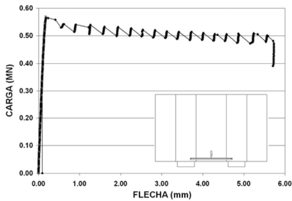
Figura 6. Curva carga-flecha. Ensayo PC-R-2.
