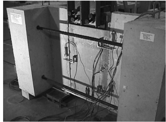
Figura 7. Configuración general del ensayo PC-R.
