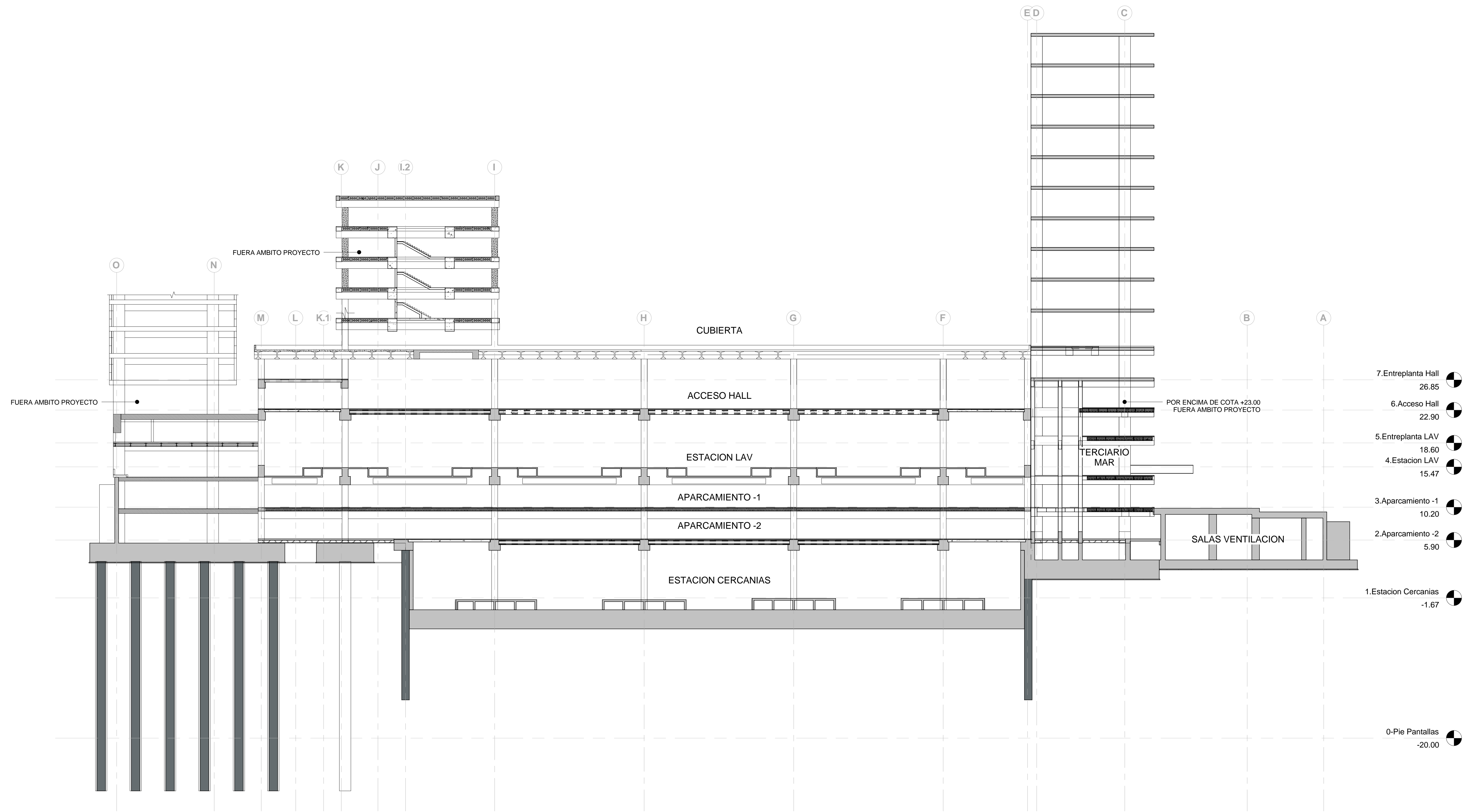
1 SECCION EJE-15 1 : 250
